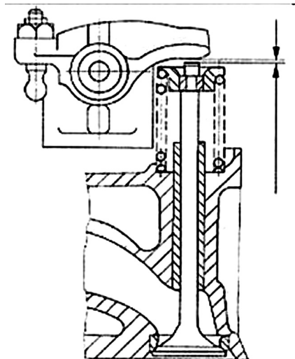
Рисунок 1 Регулировка клапанного зазора
