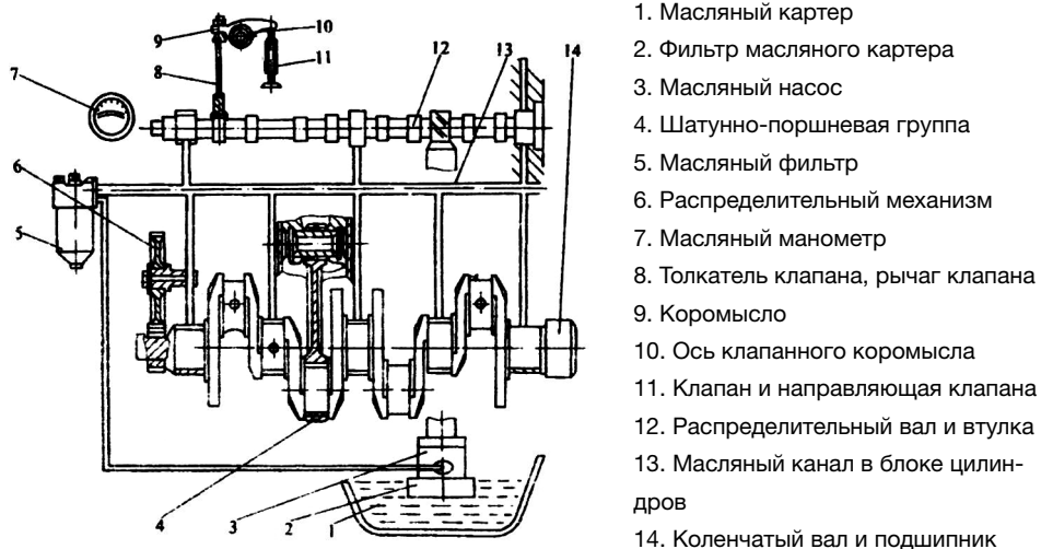
Рисунок 11 Система смазки
