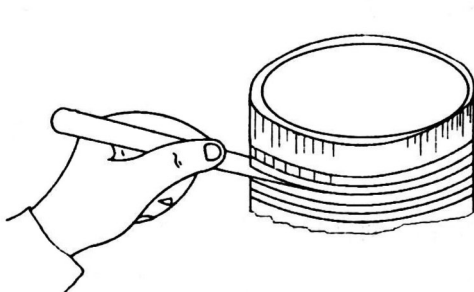
Рисунок 8. Измерение бокового зазора поршневого кольца
